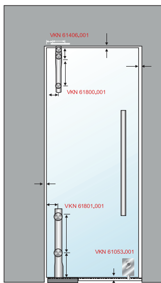
Bản lề sàn VVP/VICKINI
